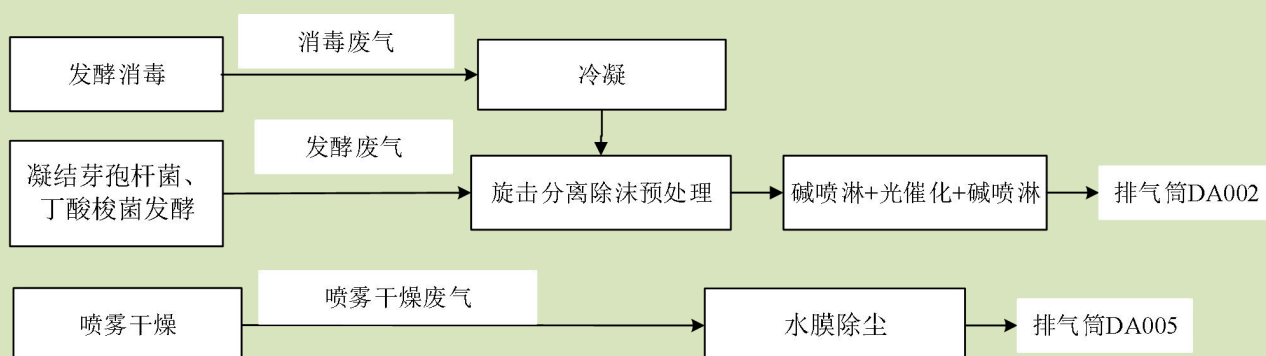
图 4.5-1 项目废气处理示意图
