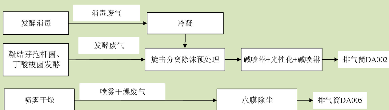
图 7.2-1 本项目废气处理工艺流程图
