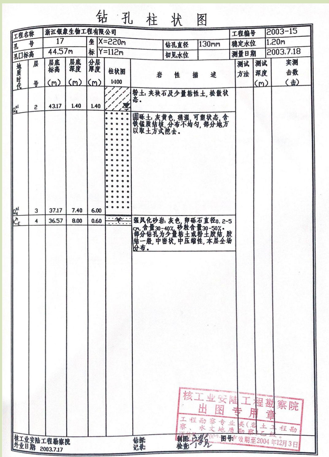
图 6.5-1 场地典型钻孔柱状图
