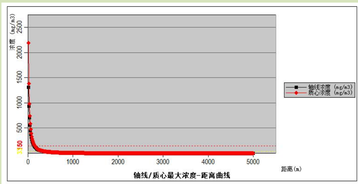
图 6.7-3 盐酸泄漏最大影响浓度与距离关系图
